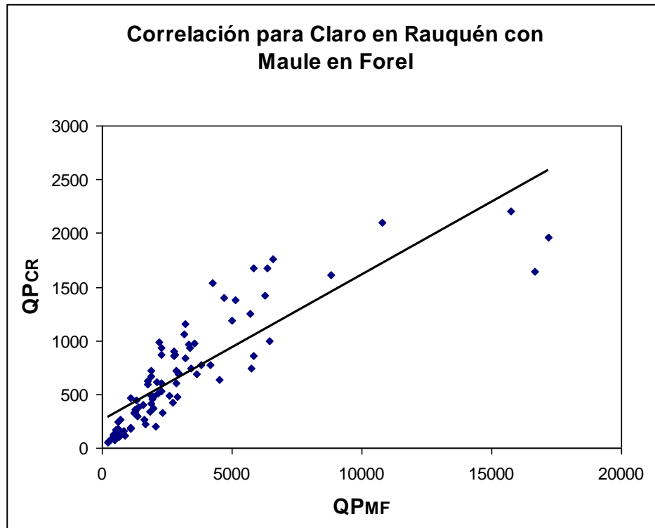
Figura 1. Diagrama de dispersión para el caudal punta de la estación aguas arriba ( QP_{CR} ) y el caudal punta de la estación aguas abajo ( QP_{MF} ).
