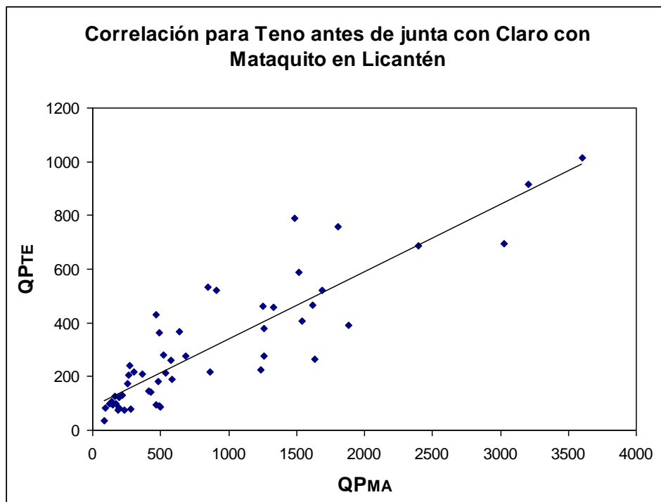
Figura 10. Diagrama de dispersión para el caudal punta de la estación aguas arriba ( QP_{TE} ) y el caudal punta de la estación aguas abajo ( QP_{MA} ).
