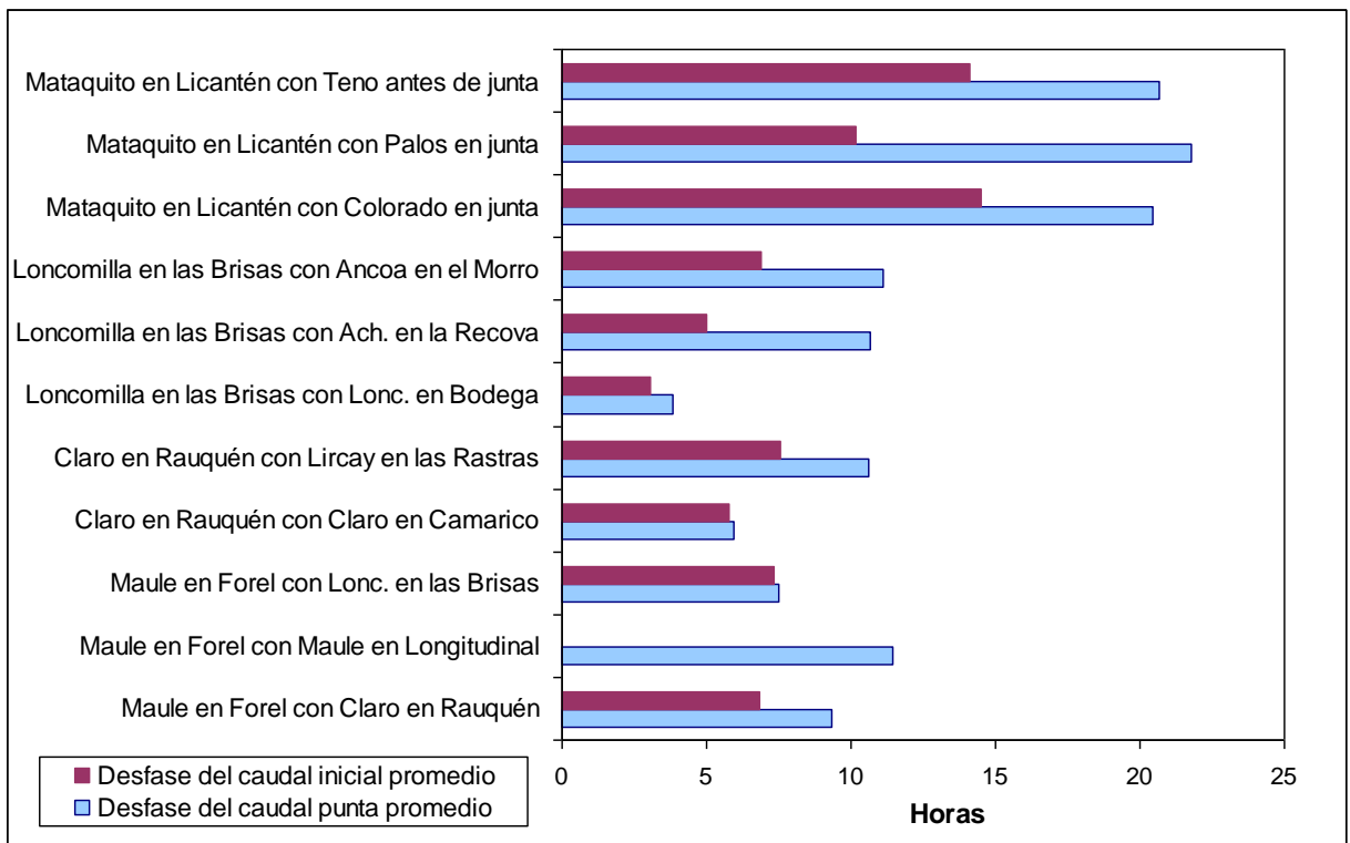
Figura 20. Desfases promedio para las relaciones entre estaciones.
