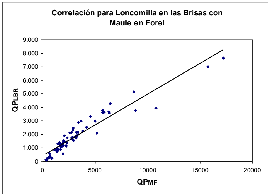
Figura 2. Diagrama de dispersión para el caudal punta de la estación aguas arriba (Q PLBR ) y el caudal punta de la estación aguas abajo (Q PMF ).
