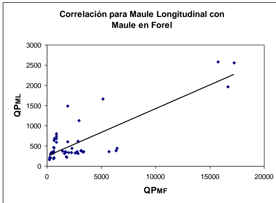
Figura 3. Diagrama de dispersión para el caudal punta de la estación aguas arriba (Q PML ) y el caudal punta de la estación aguas abajo (Q PMF ).
