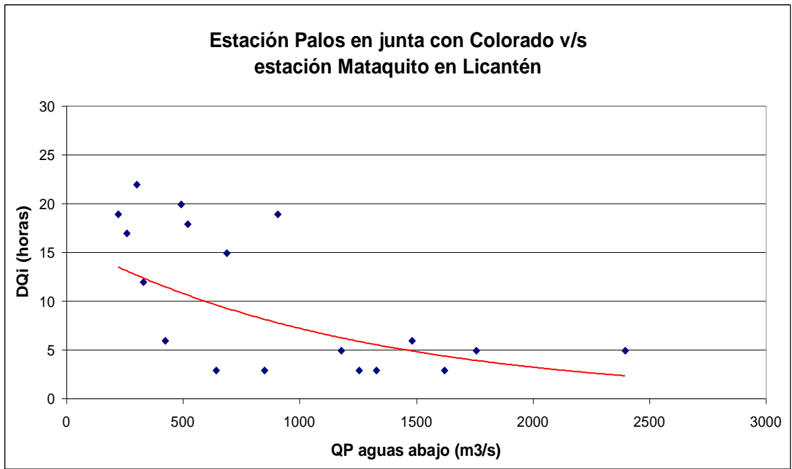
Figura 19. Relación entre el desfase del caudal inicial con los caudales punta de la estación Mataquito en Licantén.
