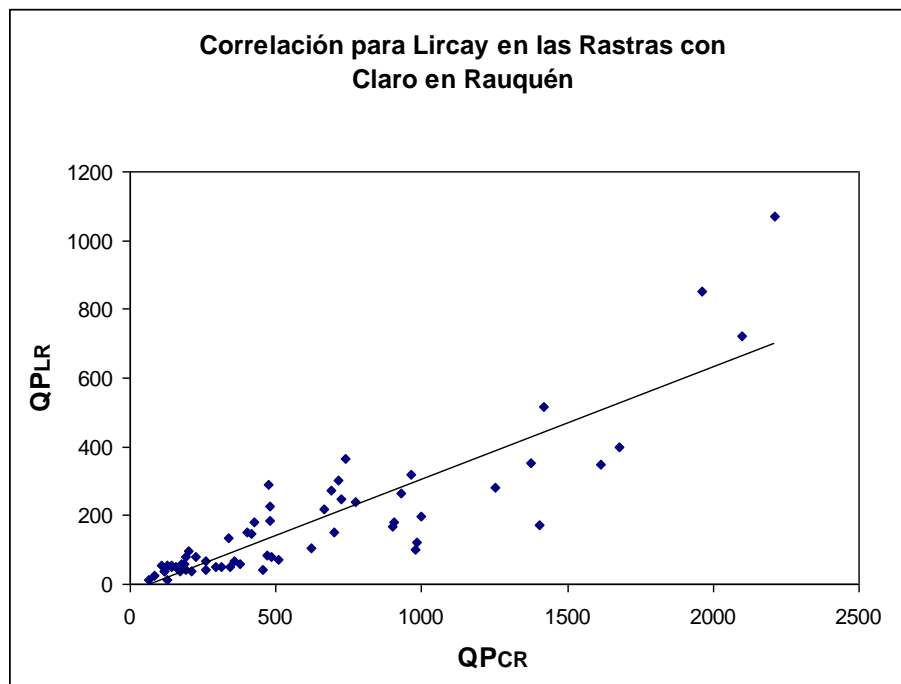
Figura 5. Diagrama de dispersión para el caudal punta de la estación aguas arriba ( QP_{LR} ) y el caudal punta de la estación aguas abajo ( QP_{CR} ).
